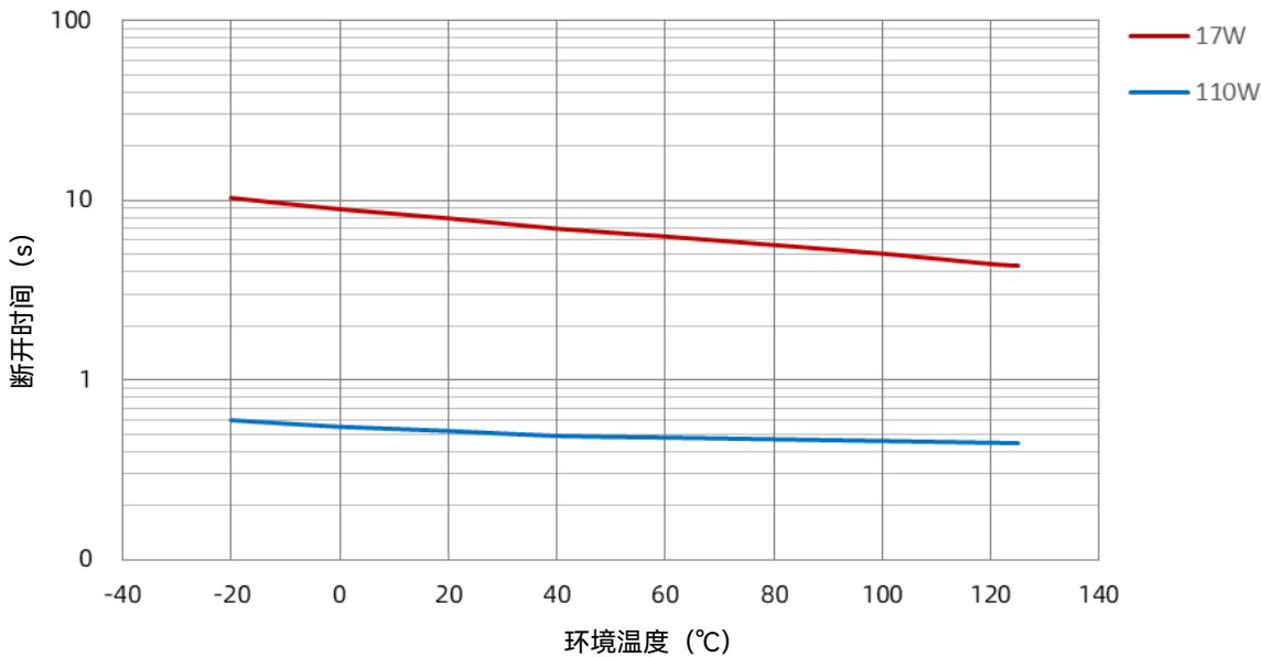
SHP 30 A 功率-温度曲线
