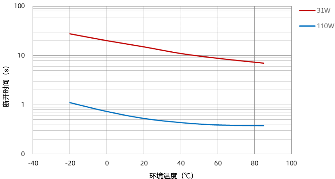
SHP 75 A 功率-温度曲线
