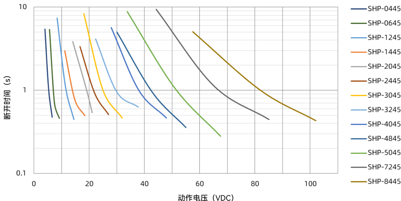
SHP 45 A 受控熔断时间曲线
