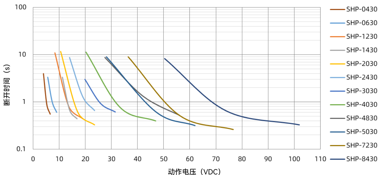
SHP 30 A 受控熔断时间曲线
