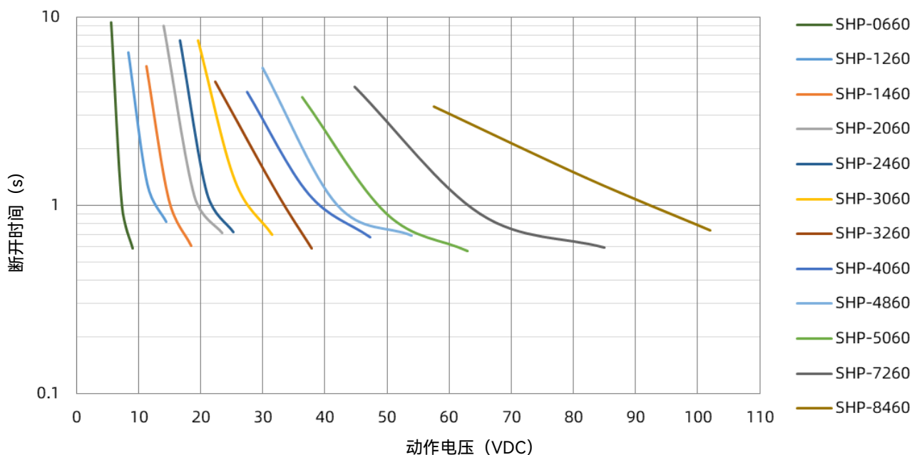
SHP 60 A 受控熔断时间曲线
